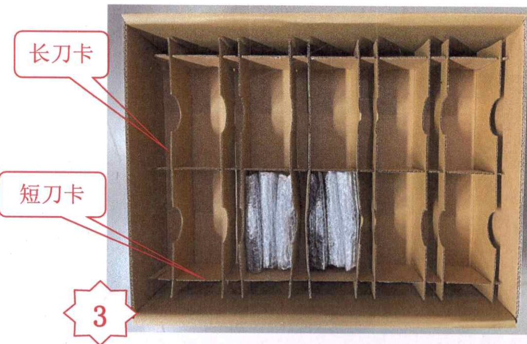
图三, 每箱两层包装, 在底部、中层、顶部各放一块隔板共三块平隔板。
